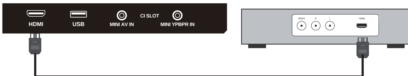
Підключення HDMI
