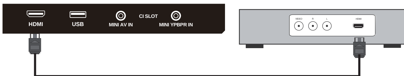
Подключение HDMI
